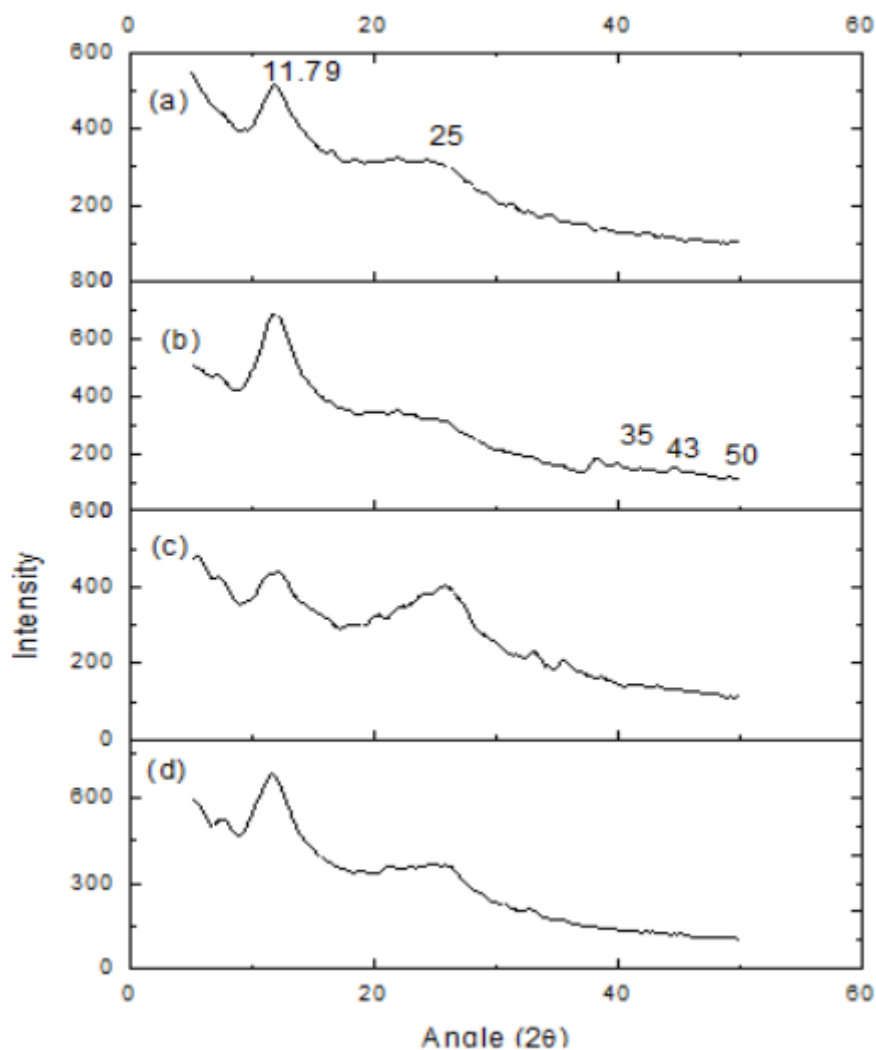
Figure1.XRD Spectrum of (a) PPy (b)PPy/MWCNT (10wt%) (c) PPy/MWCNT (5wt%) (d) PPy/MWCNT (3wt%) composites
